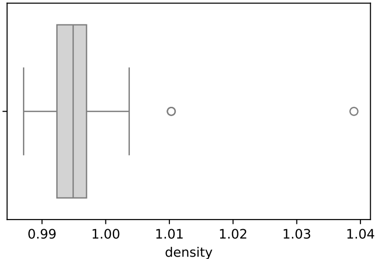
Box-plot Incondicional - density
